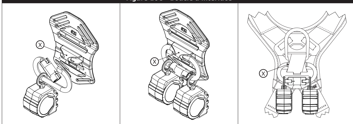
Figure 10C - Boucle d'interface
