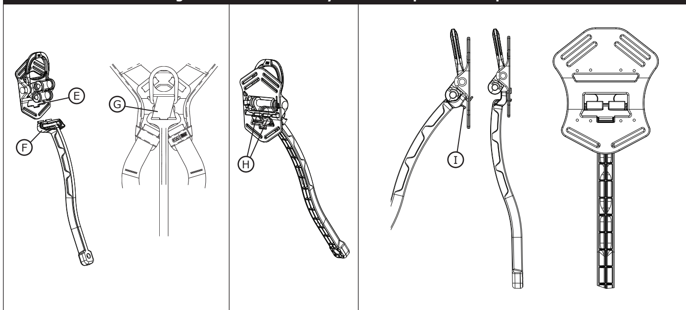
Figure 11 - Fixation du système de répartition du poids
