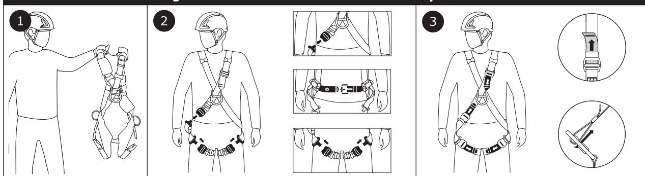
Figure 6B - Enfillement du harnais de style croisé
